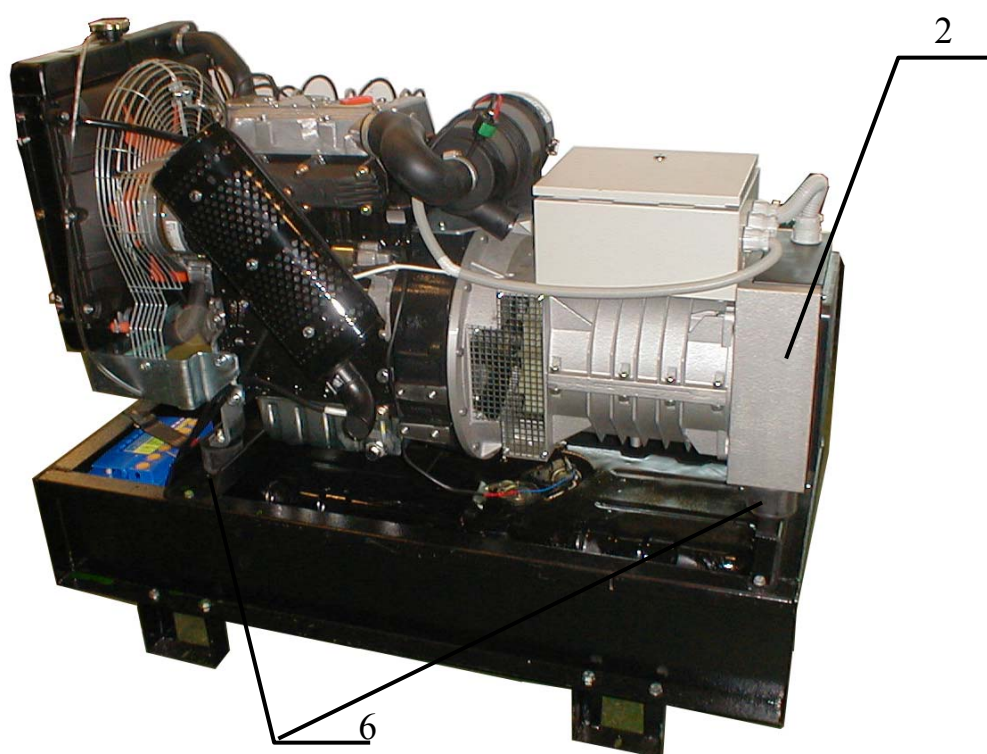
Рис. 3а. Вид со стороны глушителя двигателя LDW1603
