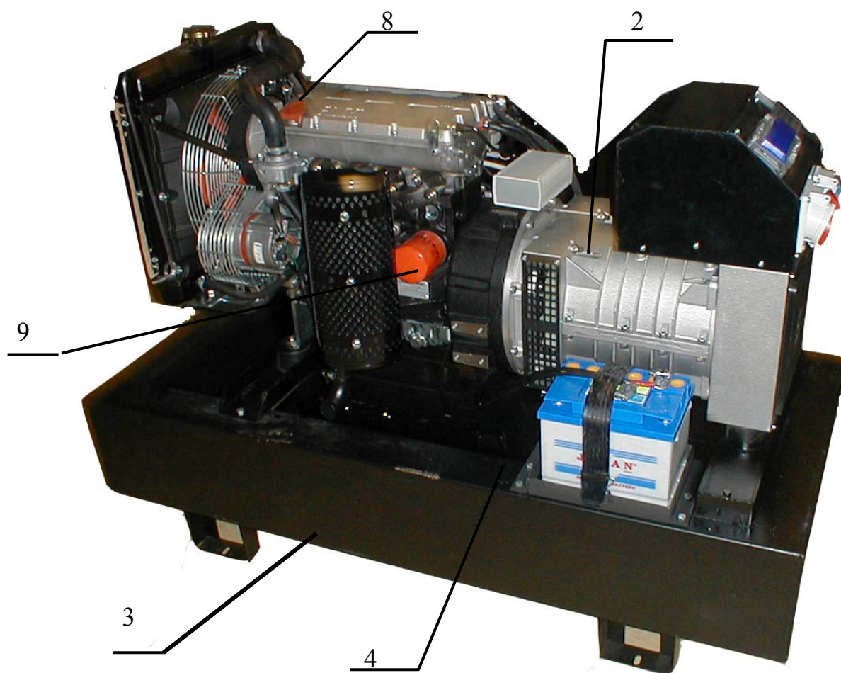
Рис. 2а. Вид со стороны размещения аккумулятора
