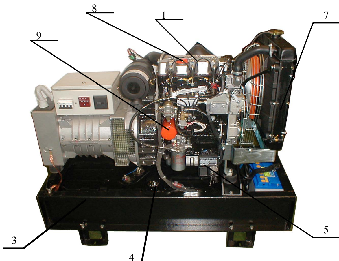
Рис. 3. Вид с обслуживаемой стороны двигателя LDW1603
