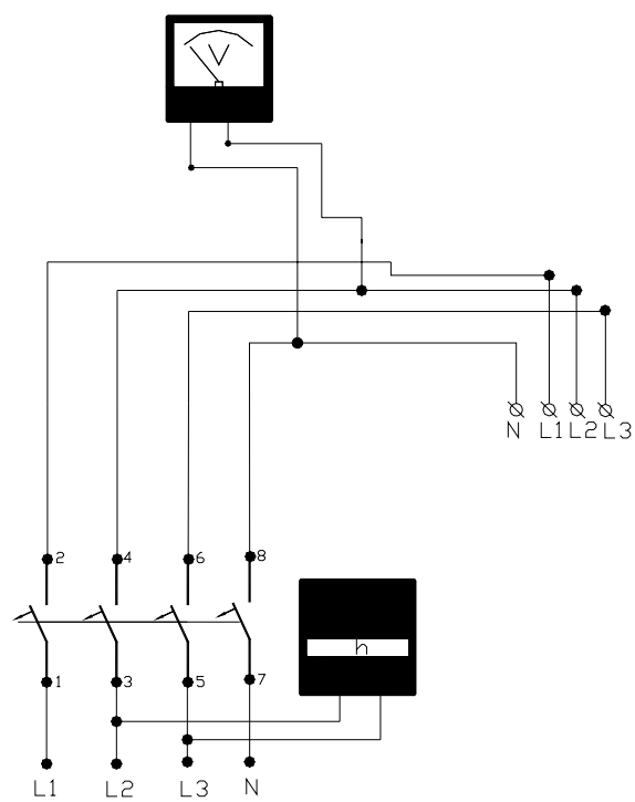
Рис. 5а. Электрическая схема силовая электрогенератора с двигателем Lombardini LDW1603
