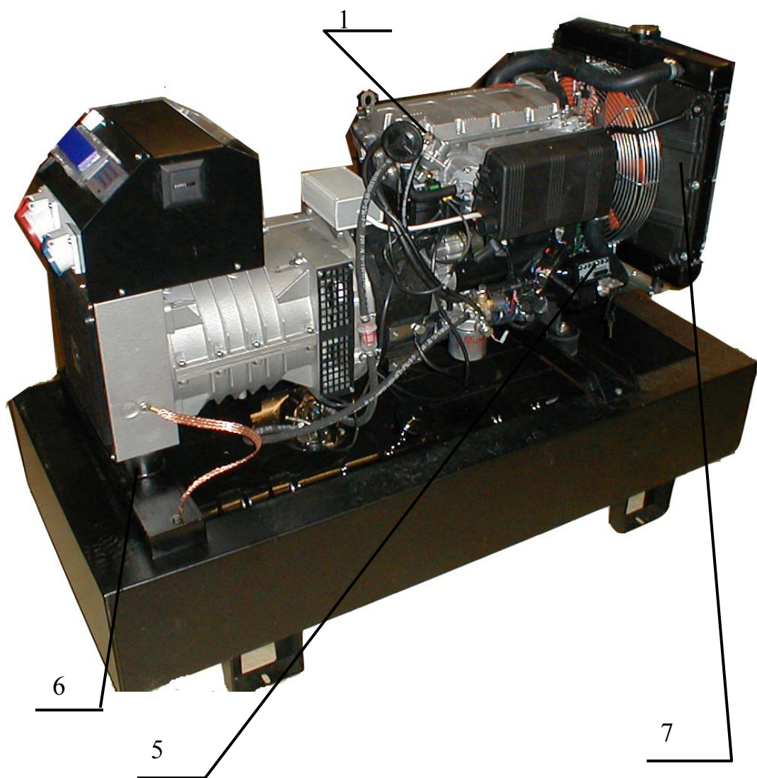
Рис. 2. Вид с обслуживаемой стороны двигателя
